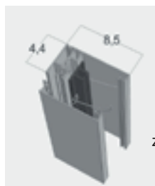
Cassonetto ispezionabile
